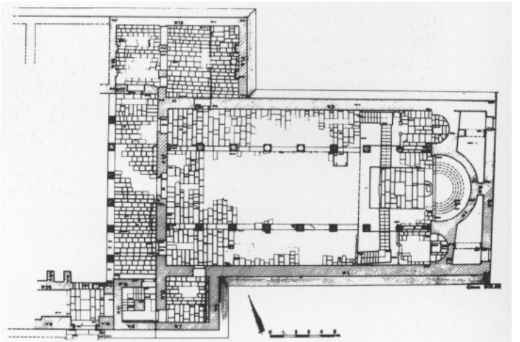
רחובות בנגב; תכנית הכנסייה הצפונית
